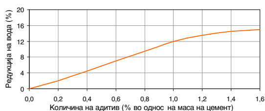
Редукуција на вода согласно EN 480-1 и EN 934-2, Табела 2.
